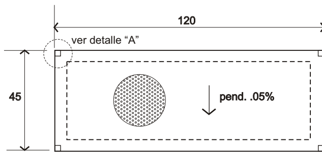
VISTA SUPERIOR
