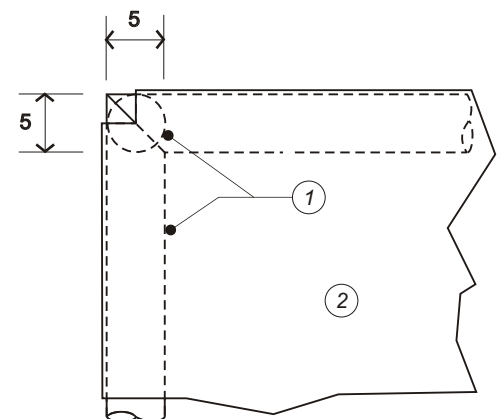
DETALLE CONSTRUCTIVO "A"
