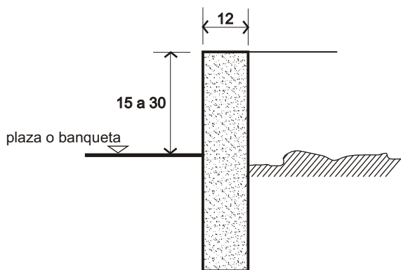
DETALLE CONSTRUCTIVO
