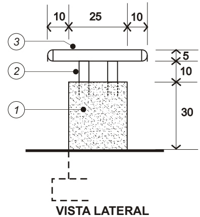
VISTA LATERAL
