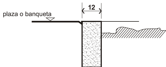
DETALLE CONSTRUCTIVO
