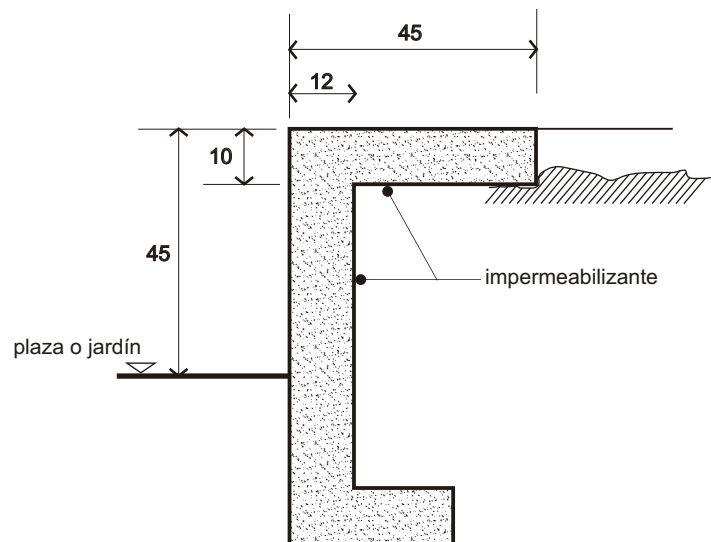
DETALLE CONSTRUCTIVO
