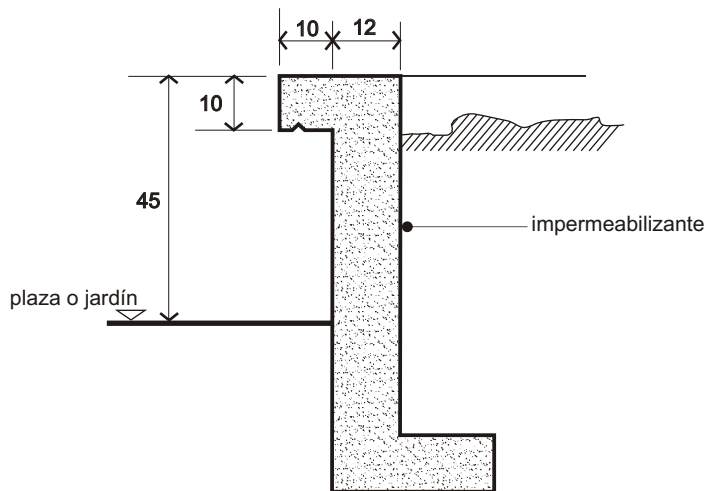
DETALLE CONSTRUCTIVO
