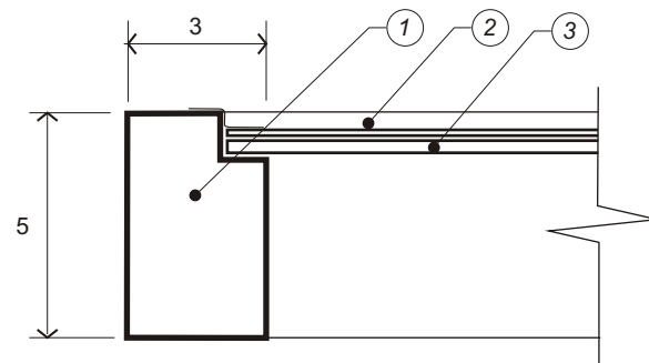
DETALLE CONSTRUCTIVO
