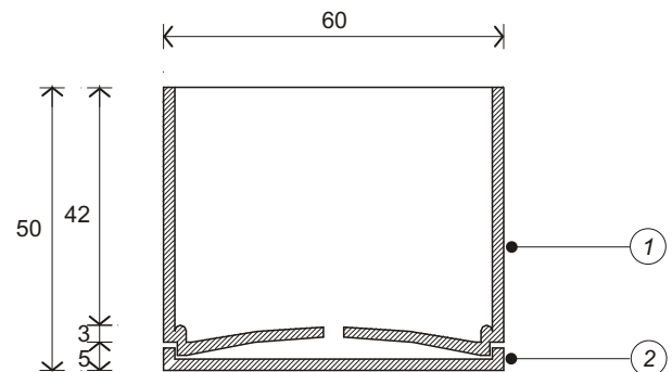
CORTE
