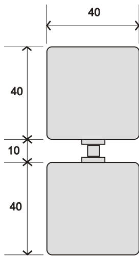
VISTA SUPERIOR
