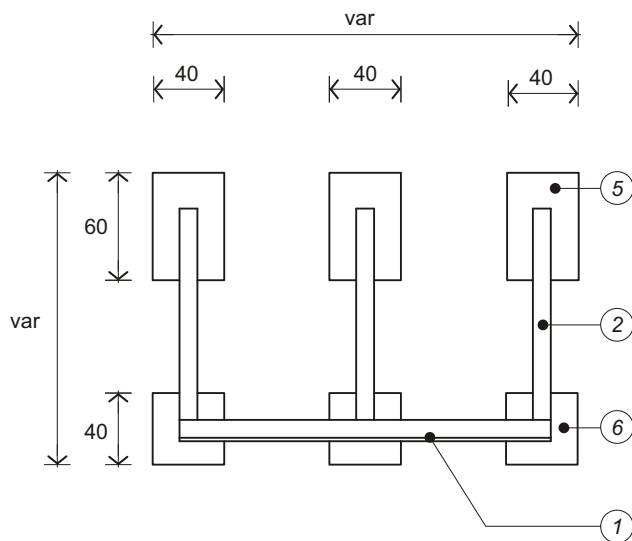
VISTA SUPERIOR
