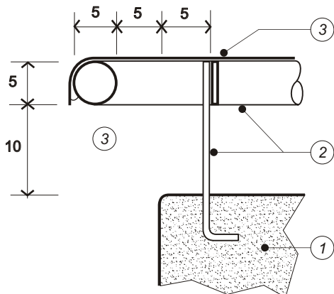
DETALLE CONSTRUCTIVO "B"
