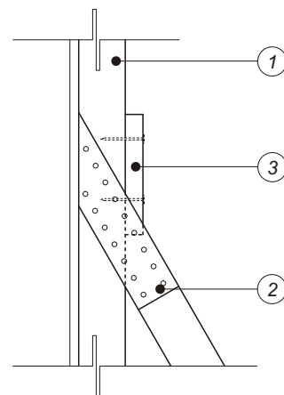
DETALLE CONSTRUCTIVO
