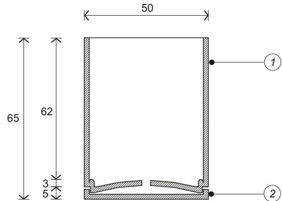
CORTE
