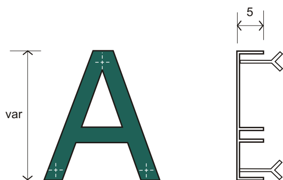
DETALLE DE ANCLAJE DE LETRERO
