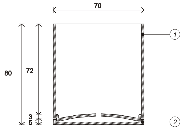
CORTE A-A
