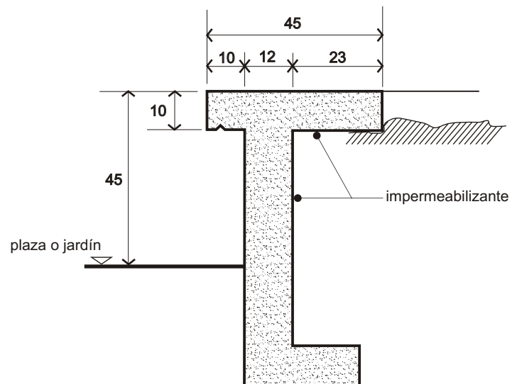
DETALLE CONSTRUCTIVO
