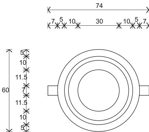
VISTA SUPERIOR
