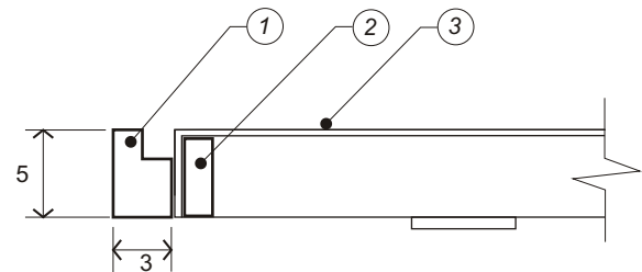
DETALLE CONSTRUCTIVO
