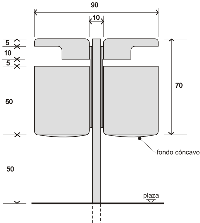
VISTA LATERAL
