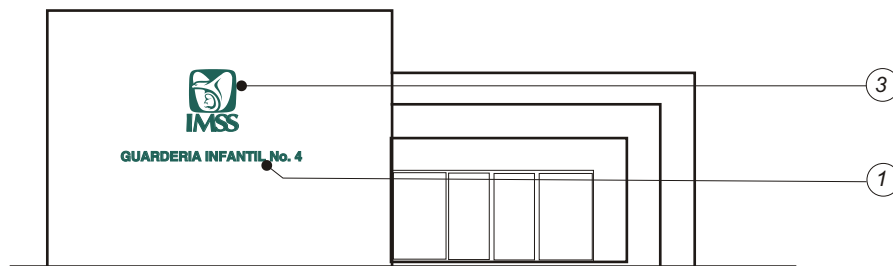
VERTICAL SIMETRICO
