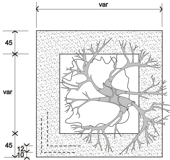
VISTA SUPERIOR
