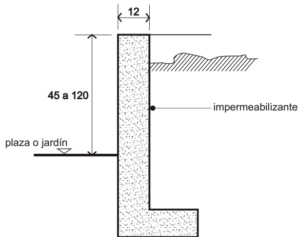
DETALLE CONSTRUCTIVO
