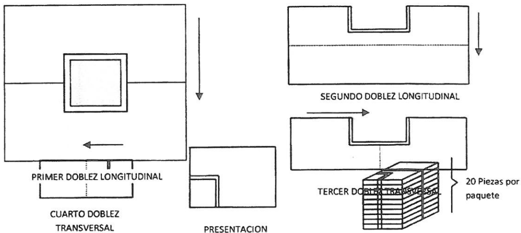
BULTO EMPALMADO ó EMPAQUETADO
