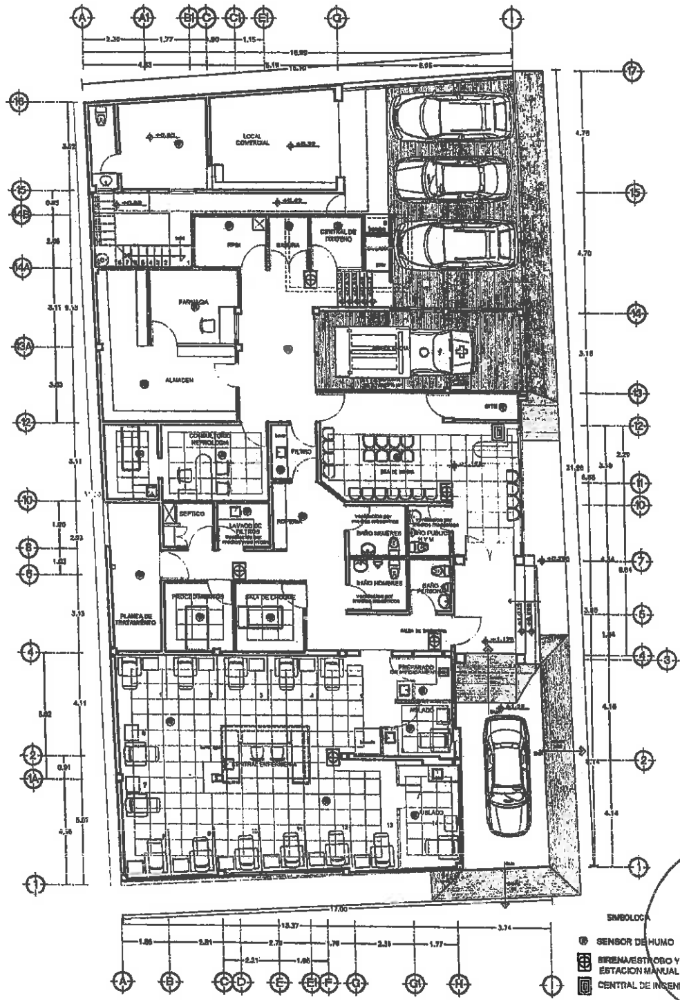
Planta Baja Detector de Humo
