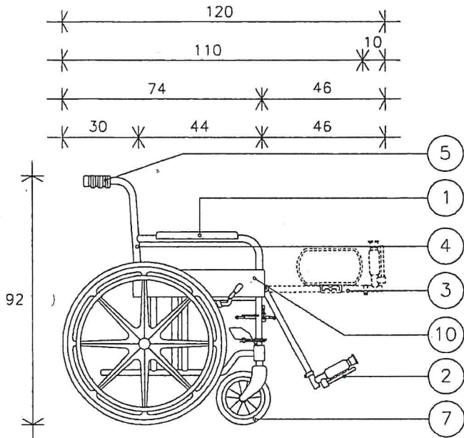
VISTA LATERAL
