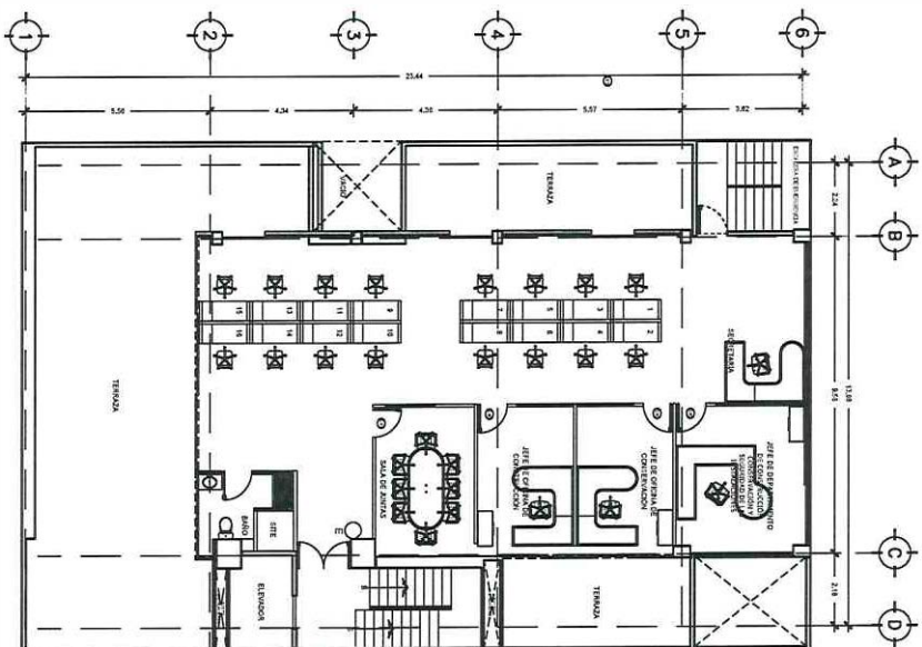
NOVENO NIVEL
