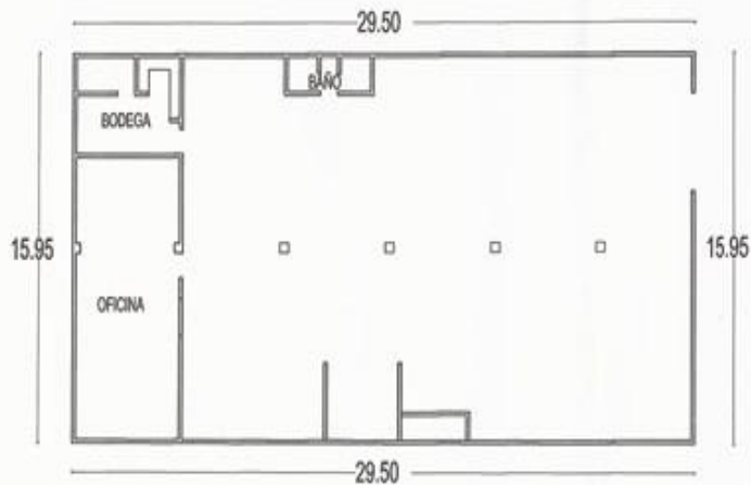
PLANTA ARQUITECTONICA
