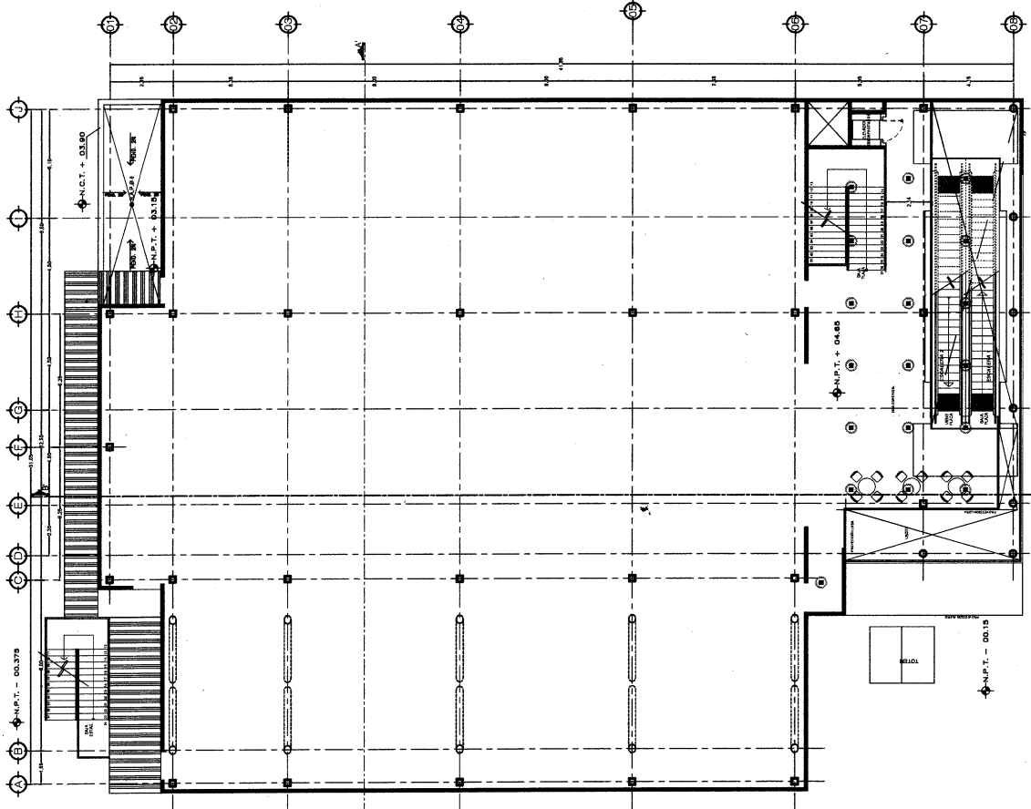
PLANO ARQUITECTÓNICO - PLANTA ALTA ÁREA : 1,268.01 M2 ESC: 1:100
