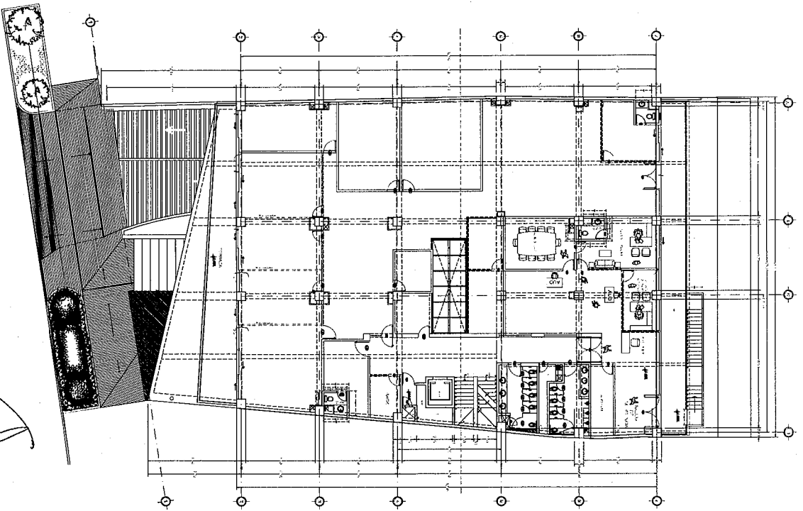
EDIFICIO SAT - PLANTA 3º NIVEL AREA TOTAL 3º NIVEL : 965,96 M2 AREA DE ARRENDAMIENTO : 60,69 M2
