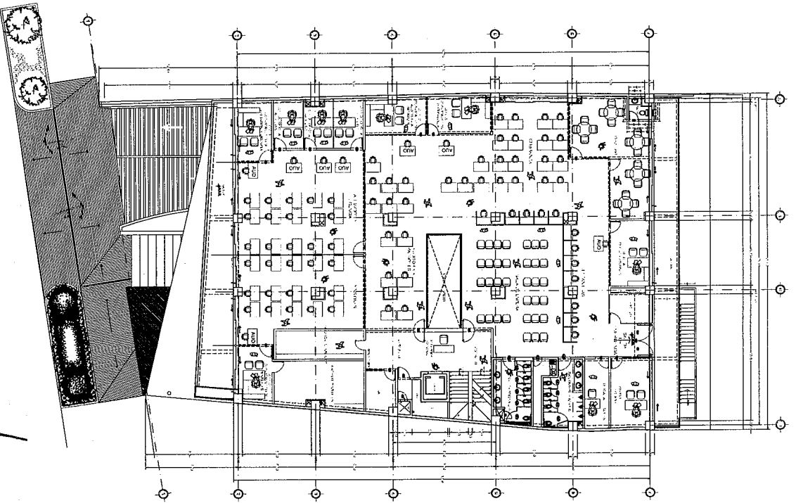
EDIFICIO SAT - PLANTA 2º NIVEL AREA TOTAL 2º NIVEL : 965,96 M2
