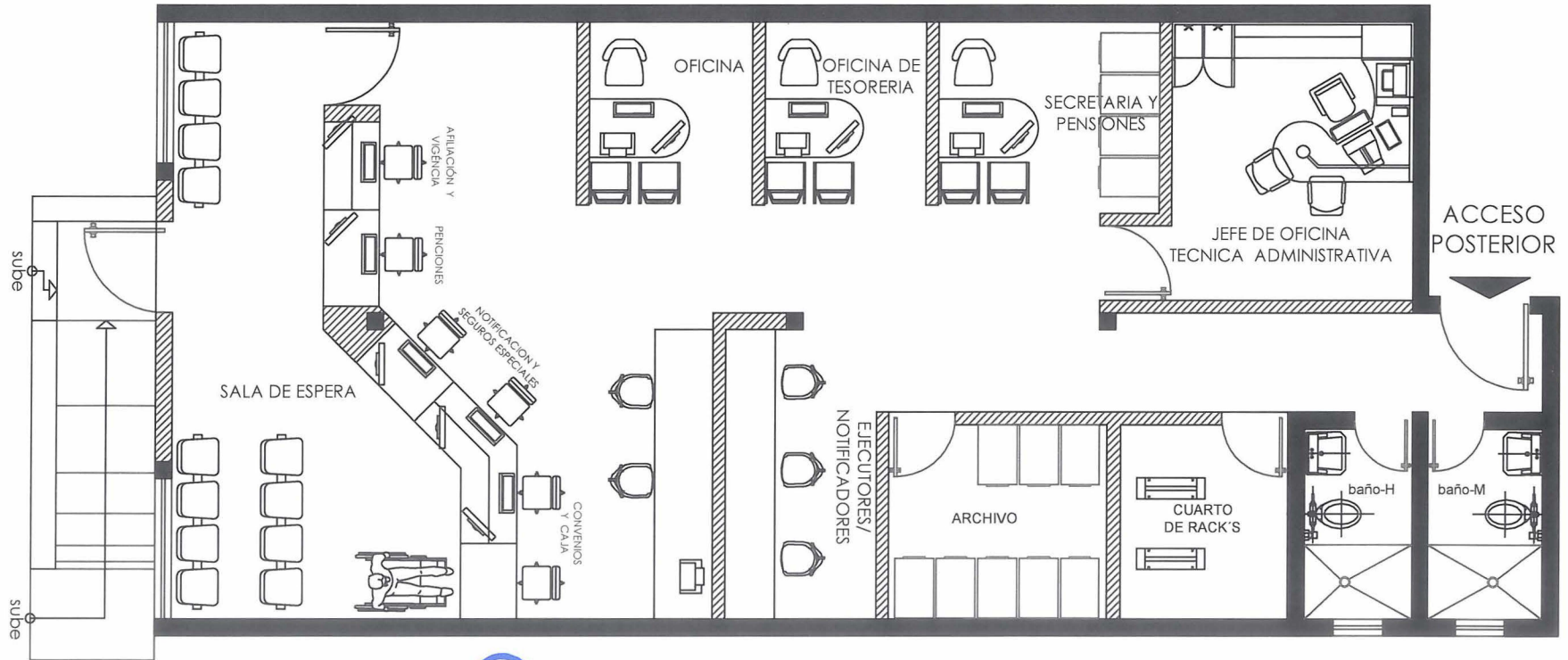
PLANTA ARQUITECTONICA ÁREA: 147.00m 2
