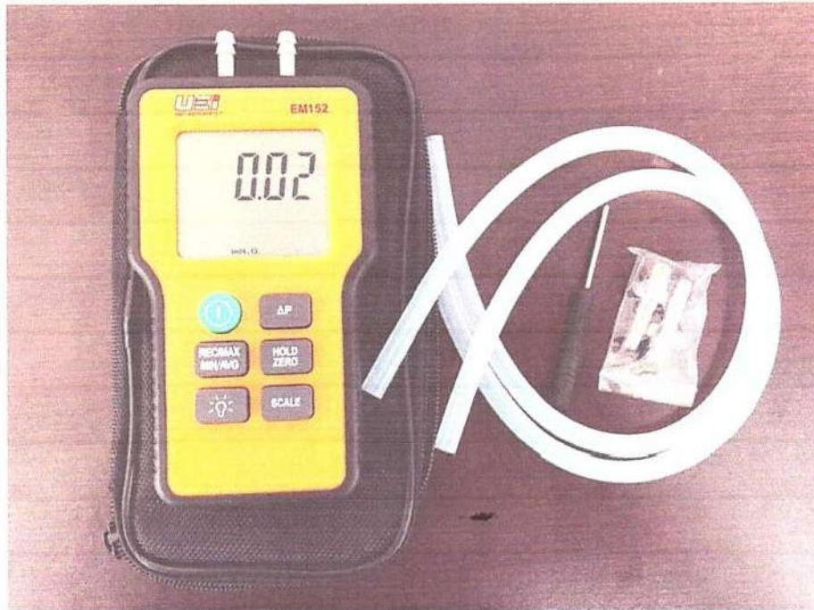
MANÓMETRO DIGITAL DE PRESIÓN DIFERENCIAL DUAL, MARCA: UEI, MODELO: EM152
