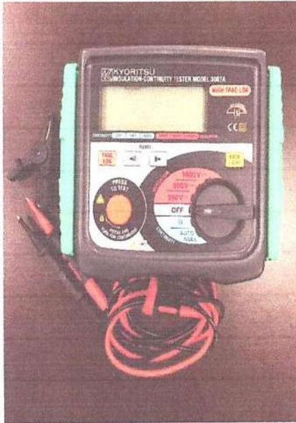
PROBADOR DE CONTINUIDAD Y AISLAMIENTO DIGITAL 250 V/500 V/1000 V, MARCA: KYORITSU, MODELO: 3007A
