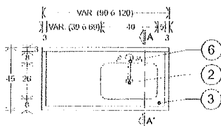
VISTA SUPERIOR
