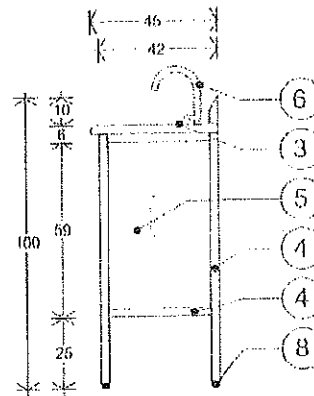
VISTA LATERAL
