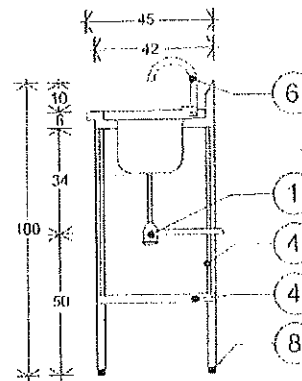
CORTE A,A'
