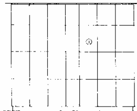
ALZADO MURO 836 100
