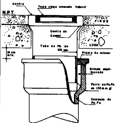
TAPON REGISTRO EN PIE DE B.A.N. y/o B.A.P.
