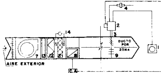
28. - UMA TIPO UNIZONA CON SERPENTIN DE AGUA REFRIGERADA Y 100% AIRE EXTERIOR
