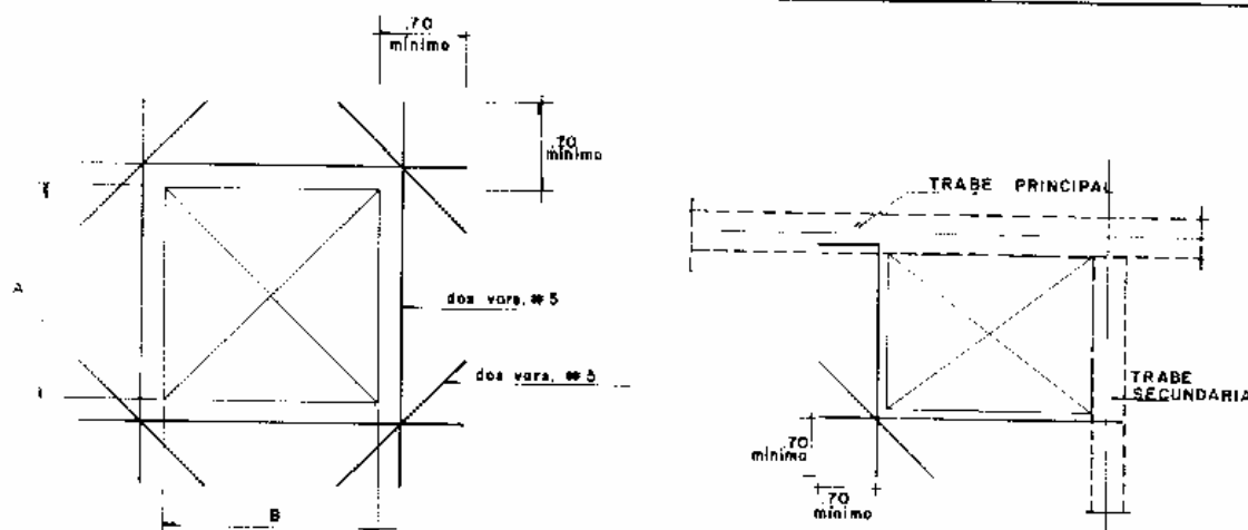
CRITERIOS DE REFUERZO PARA HUECOS
