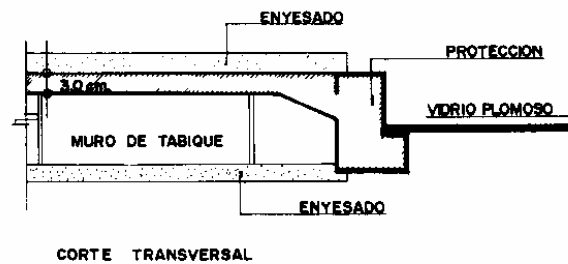
CORTE TRANSVERSAL
