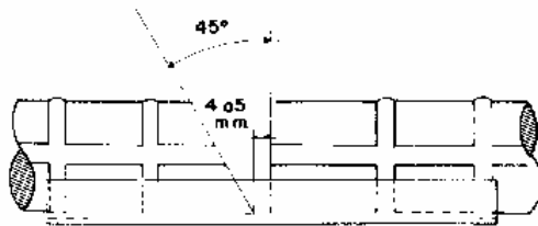
ANGULO O PLACA CURVA DE RESPALDO.
