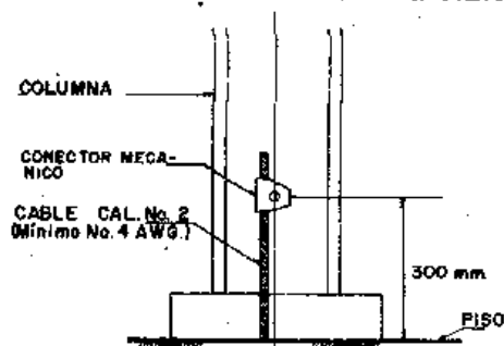
CONECTOR MECANICO CON TORNILLO PARA CABLE EN COLUMNA METALICA
