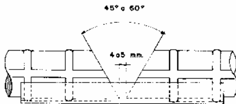
ANGULO O PLACA CURVA DE RESPALDO.
