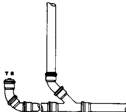
TAPON REGISTRO EN PIE DE B.A.N. y/o B.A.P.
