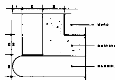
PLANTA 7.-ESQUINA DESTAZADA BOLEADA
