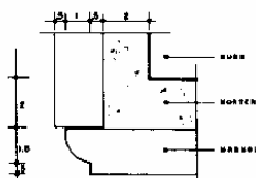
PLANTA 3.-ESQUINA C/MOLDURA
