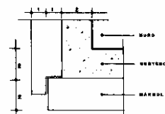
PLANTA 4.-ESQUINA CON CAJA
