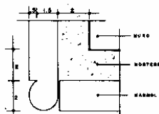
PLANTA 5.-ESQUINA CON TORO
