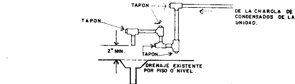
DRENAJE DE CONDENSADOS DE LAS- UNIDADES SERPENTIN VENTILADOR. (FAN AND COIL).
