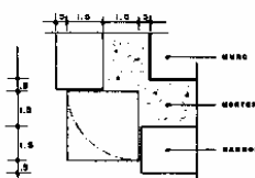
PLANTA 9.-ESQUINA CON CUADRO
