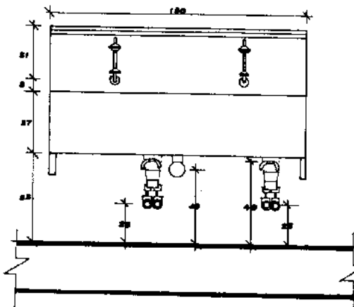
VISTA FRONTAL.
