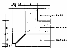
PLANTA 2.-ESQUINA a 45°
