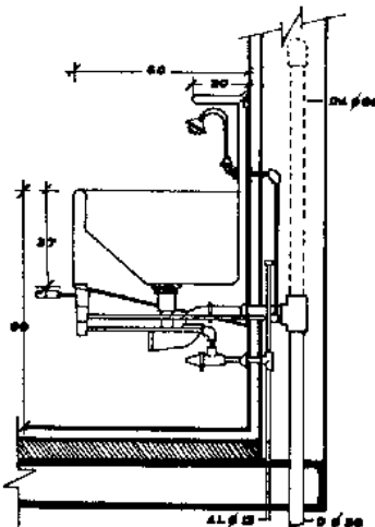
ELEVACION.
