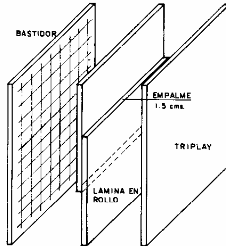
LAMINA EN ROLLOS DE 60 cm. DE ANCHO
