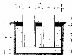
DETALLE DE CIMENTACION ALZADO E.C. 1:5
