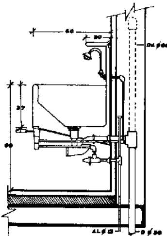
ELEVACION.
