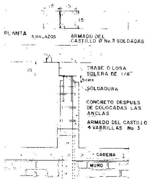
ALZADO
