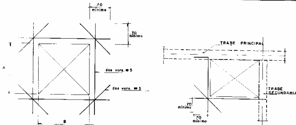
CRITERIOS DE REFUERZO PARA HUECOS
