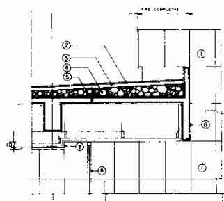
DETALLE CORTE FACHADA 43E 125
