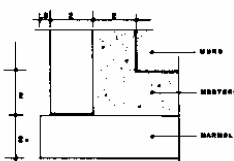
PLANTA 6ª-ESQUINA DESTAZADA
