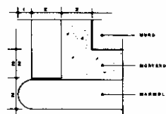
PLANTA 7ª-ESQUINA DESTAZADA BOLEADA
