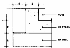
PLANTA 1ª-ESQUINA SIMPLE
