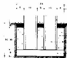
DETALLE DE CIMENTACION ALZADO E.C. 1:5
