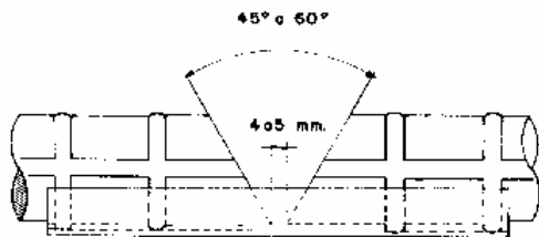
ANGULO O PLACA CURVA DE RESPALDO.
