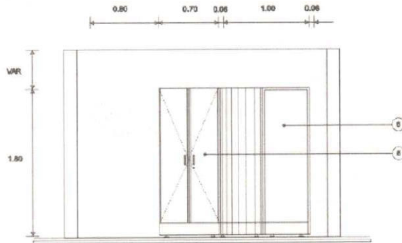
CORTE TRANSVERSAL 2
