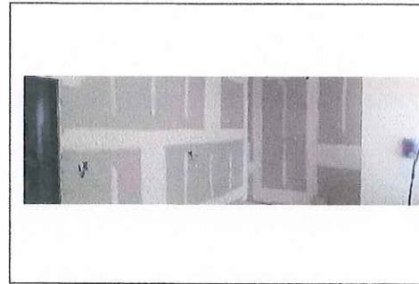
FOTO No. 5: COLOCACION DE MURO DE TABLAROCA UMF 30 ESTA FOTOGRAFIA FUE TOMADA EL DIA 25 SEPTIEMBRE 2023.
