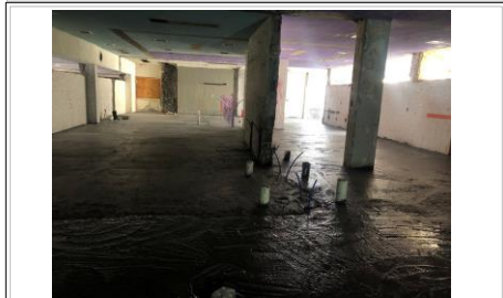
FOTO No. 7: TRABAJO TERMINADO DEL VACIADO DE LOSA ALIGERADA PARA EL CAJON DE LAS INSTALACIONES HIDROSANITARIAS.
