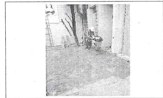
FOTO No. 6: DESCRIPCIÓN FOTOGRAFICA.- COMPACTACION DE MATERILA INERTE BAJO FIRME. ESTA FOTOGRAFIA FUE TOMADA EL DIA 31-10-2023
