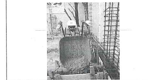
FOTO No. 9: DESCRIPCIÓN FOTOGRAFICA.- COLADO DE CONCRETO DE TRABES DE CIMENTACION . FOTOGRAFIA TOMADA EL DIA 27-10-2023
