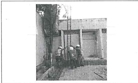
FOTO No. 4: DESCRIPCIÓN FOTOGRAFICA.- COLOCACION DE ACERO DE REFUERZO PARA COLUMNA. ESTA FOTOGRAFIA FUE TOMADA EL DIA 25-10-2023
