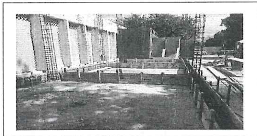
FOTO No. 7: DESCRIPCIÓN FOTOGRAFICA.- COLOCACION DE CIMBRA EN TRABES DE CIMENTACION. ESTA FOTOGRAFIA FUE TOMADA EL DIA 26-10-2023.
