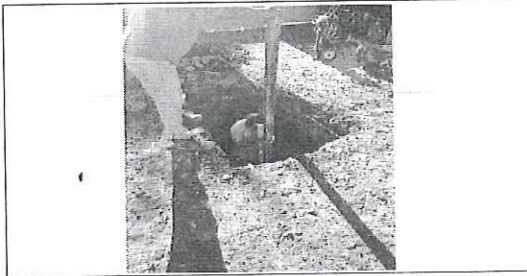
FOTO No. 1: DESCRIPCION DE FOTOGRAFIA.- PLOMEO DE ACERO DE REFUERZO PARA PEDESTALES. ESTA FOTOGRAFIA FUE TOMADA EL DIA.- 12-10-2023.
