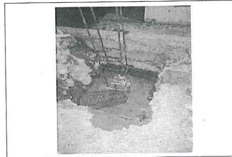
FOTO No. 5: DESCRIPCION FOTOGRAFICA.- COLADO DE CONCRETO DE ZAPATAS. ESTA FOTOGRAFIA FUE TOMADA EL DIA 13-10-2023
