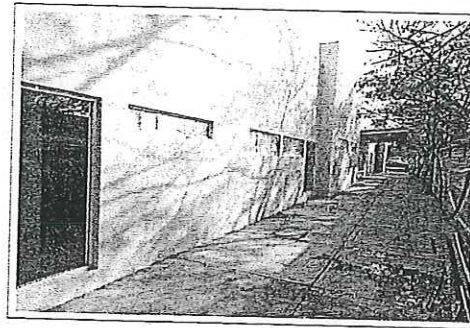
FOTO No. 5: PREPARACION DE SUPERFICIE PARA APLICACION DE PASTA COREV EN OBRA EXTERIOR ESTA FOTOGRAFIA FUE TOMADA EL DIA 31 DE ENERO DE 2024.
