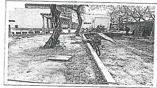
FOTO No. 3 CONFORMACION DE TERRACERIAS PARA BANQUETAS Y GUARNICIONES FOTOGRAFIA TOMADA EL DIA 31 DE ENERO DE 2024
