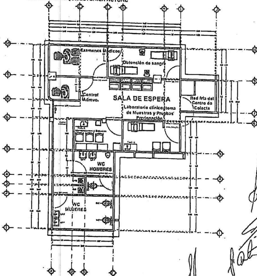
PLANTA ARQUITECTÓNICA
