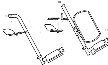
DETALLE DE DESCANSAPIES Y DETALLE DE ELEVAPIERNAS
