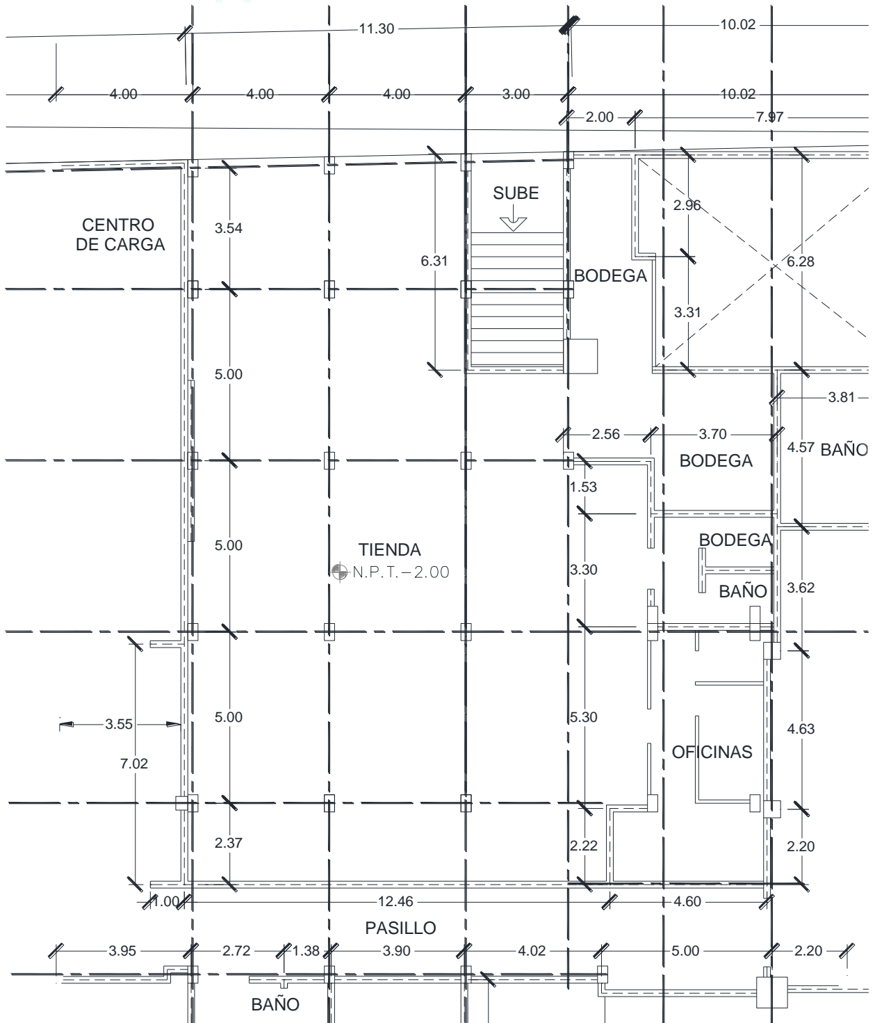
PLANO DEL DESPLANTE DEL INMUEBLE
