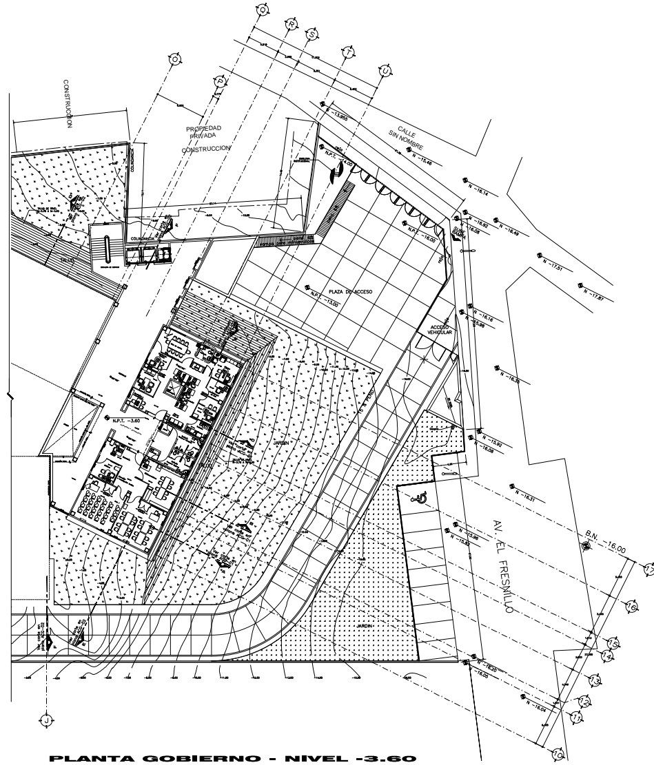
PLANTA GOBIERNO - NIVEL -3.60
