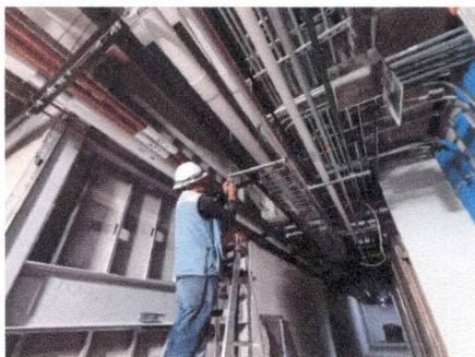
Colocación de cableado estructural en pasillo de cirugía N2
