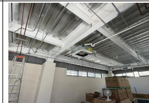
INSTALACION DE EQUIPO DE AIRE ACONDICIONADO
