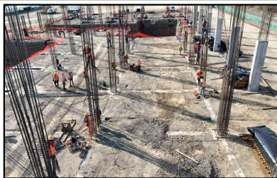
Trabajos de habilitado de acero para columnas del
