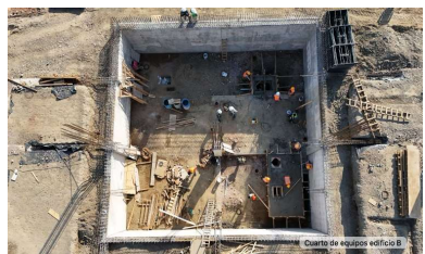
Trabajos de colado de tapas de cisternas en cuarto de equipos de Edificio "B".
