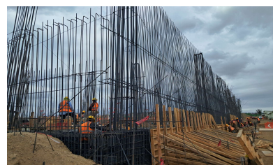
Trabajos de habilitado de acero para muro de contención del edificio "F".
