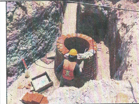
CONSTRUCCIÓN DE POZOS DE VISITA PARA RED SANITARIA
