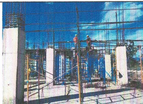
HABILITADO DE ACERO EN TRABES PB EDIF. "C"
