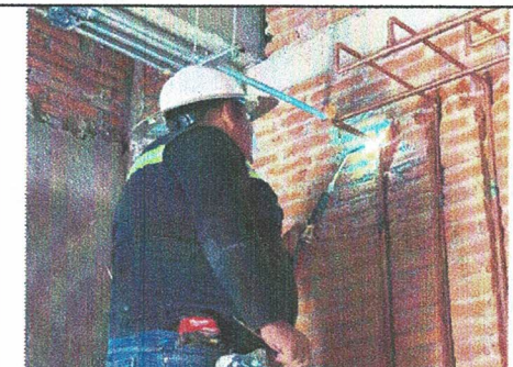
SOLDADURA EN BAJADA DE TOMAS MURALES SALA DE PROCEDIMIENTOS N-1 EDIF. "A"
