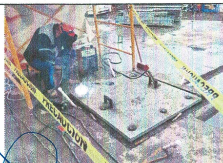
SOLDADURA EN PLACA BASE PB VESTÍBULO
