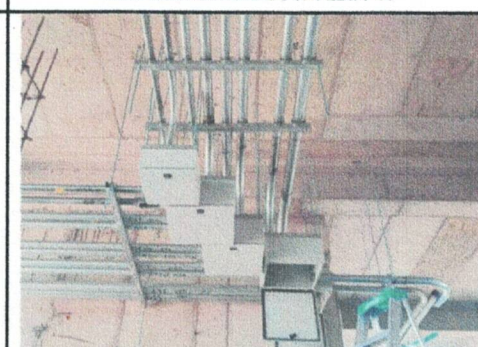
INSTALACIÓN DE CAJAS HIMEL N-2 EDIF. "B"
