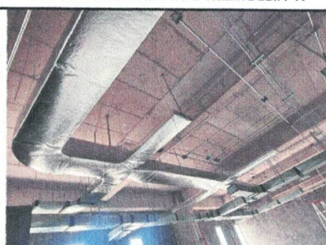
FORRO EN DUCTOS DE AIRE ACONDICIONADO N-1 EDIF. "A"
