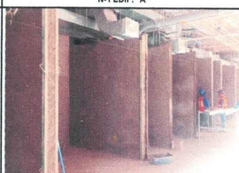
REPELLADO EN MUROS PB EDIF. "B"
