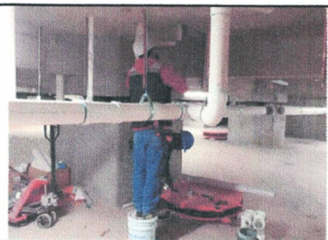
CANALIZACIÓN DE TUBERÍA DE INSTALACIÓN HIDROSANITARIA N-3 EDIF. "B"
