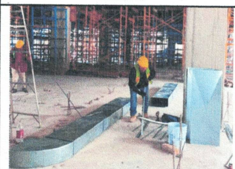
HABILITADO DE DUCTOS PB EDIF. "D"
