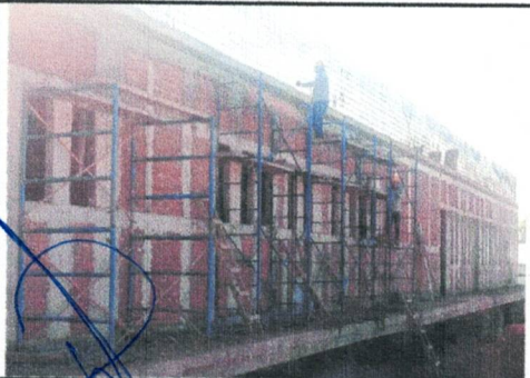
COLOCACIÓN DE CIMBRA EN DALAS Y CASTILLOS PB EDIF. "D"
