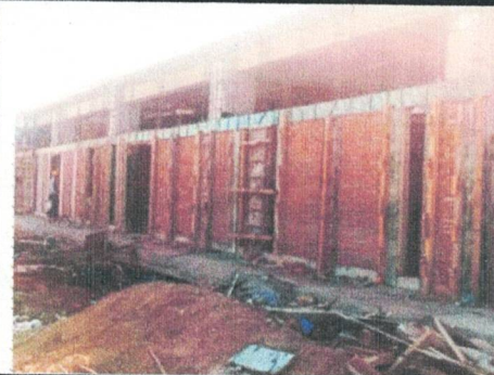
COLOCACIÓN DE CIMBRA EN DALAS Y CASTILLOS PB EDIF. "E"
