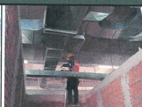
HABILITADO DE DUCTOS PB EDIF. "C"
