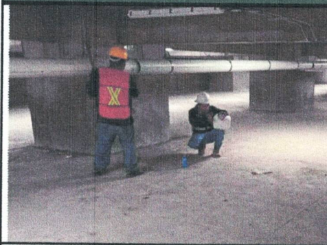
CANALIZACIÓN DE TUBERÍA DE INSTALACIÓN SANITARIA SEMISÓTANO EDIF. "C"
