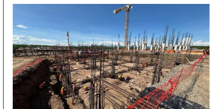
Trabajos de armado de acero de refuerzo en cimentación
