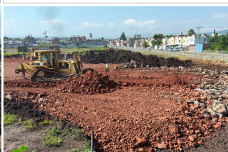
Conformación de material de filtro para plataforma en estacionamiento lado Sur -Este.
