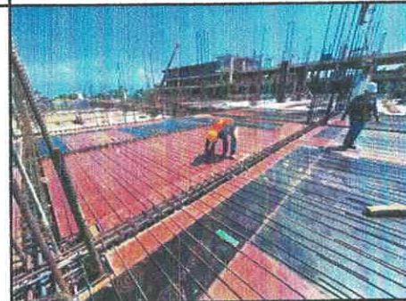
ARMADO DE PARILLA EN LOSA DE N-1 EDIF. "C"
