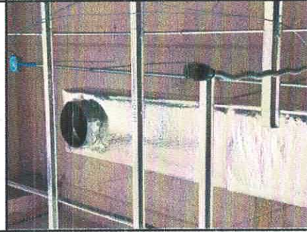
COLOCACIÓN DE CUELLOS FLEXIBLES PARA REJILLAS PB EDIF. "A"
