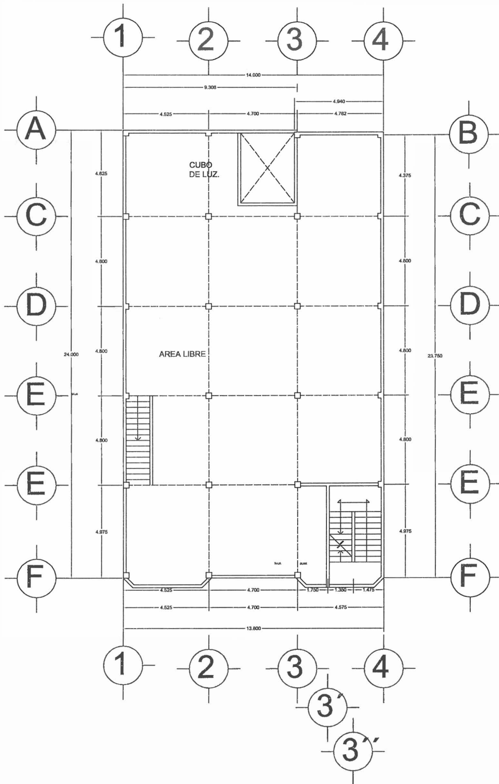
PLANTA 1° NIVEL
