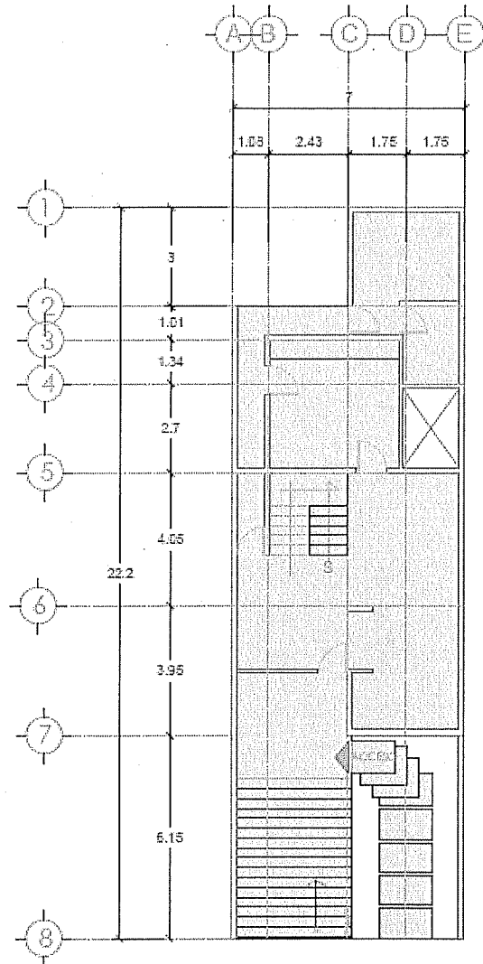
PLANTA ARQUITECTÓNICA
