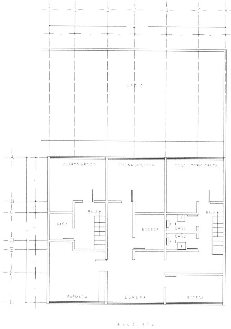
PLANTA ARQUITECTÓNICA ALTA DE LA U.M.F. No.6
