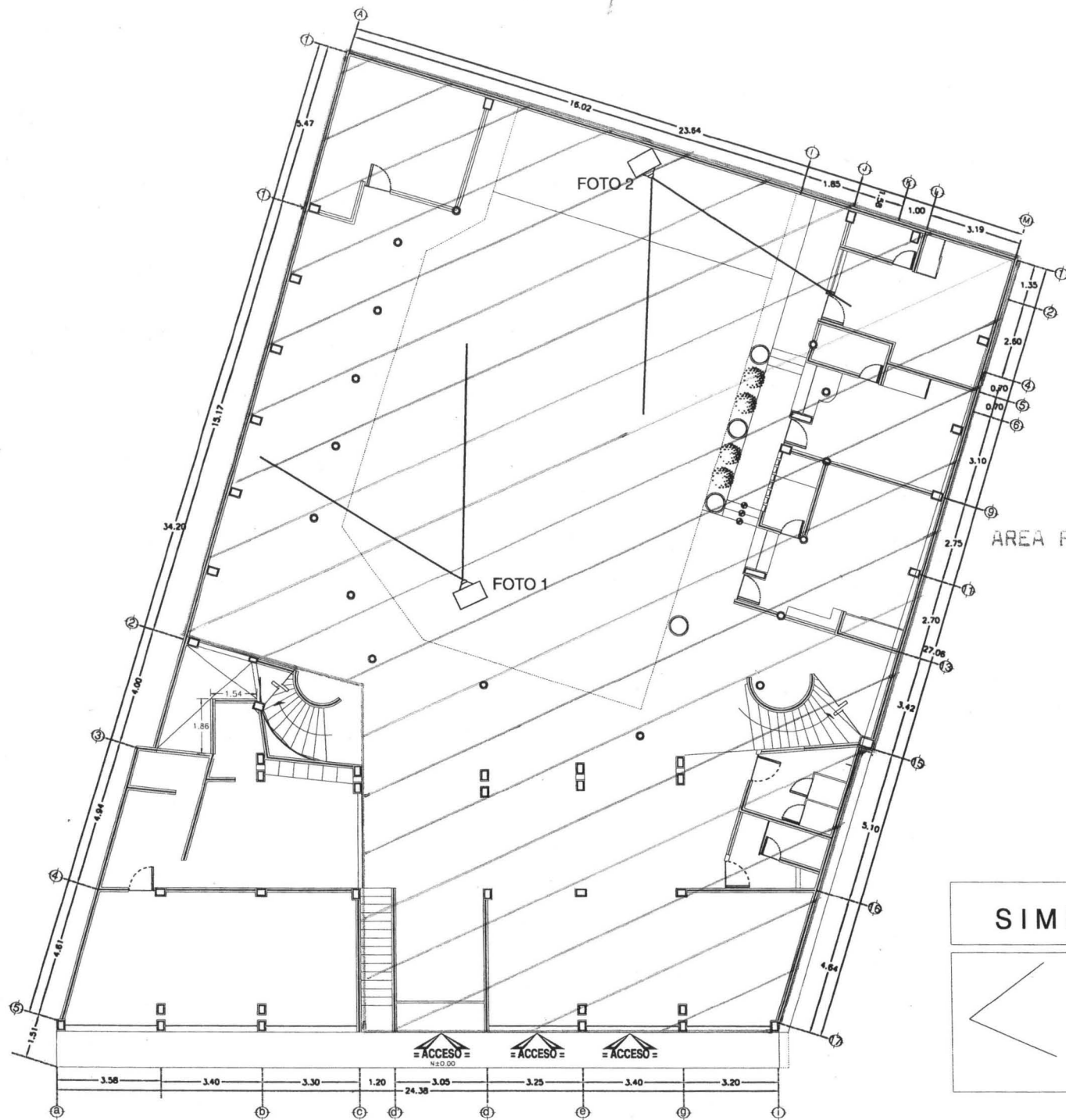
PLANTA ARQUITECTONICA BAJA.
