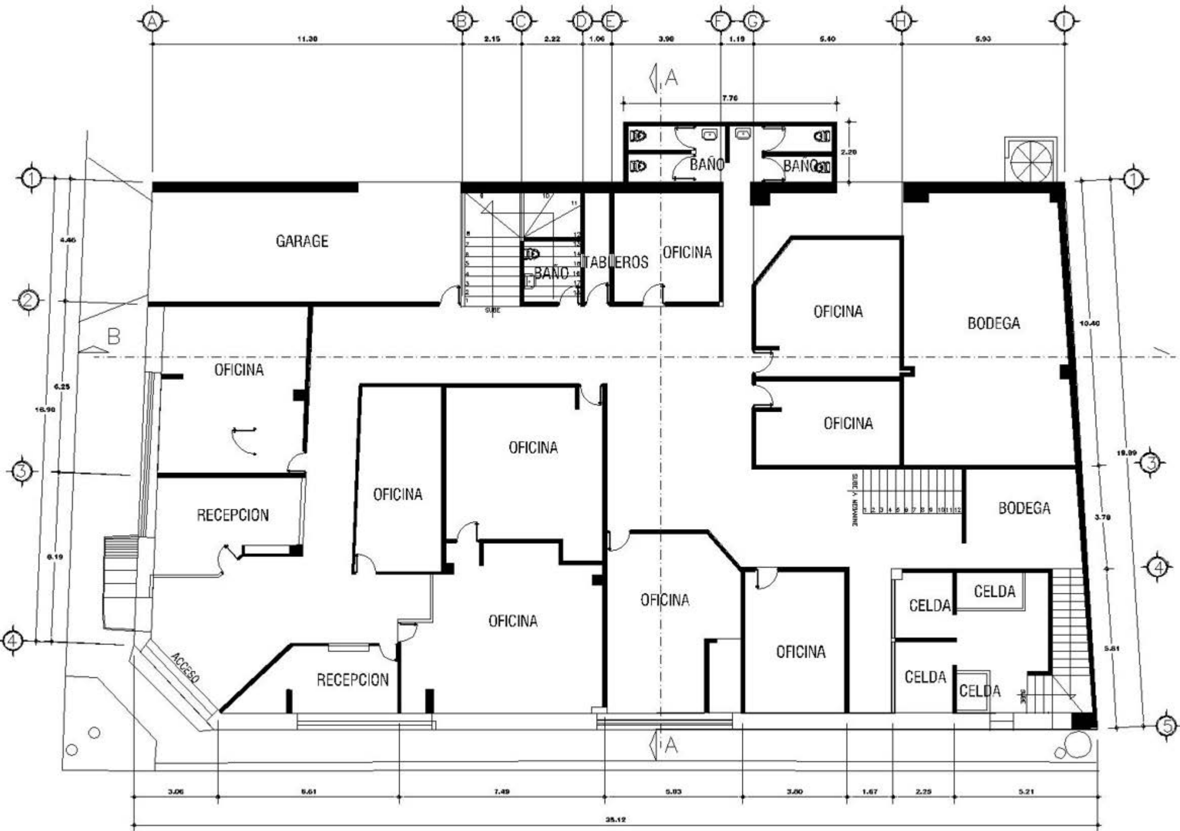
PLANTA ARQUITECTONICA ESTADO PLANTA BAJA
