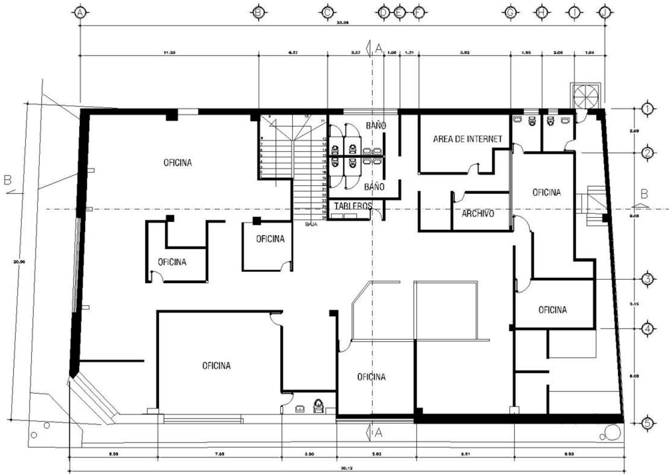
PLANTA ARQUITECTONICA ESTADO PLANTA ALTA
