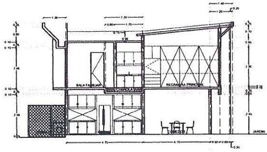
CORTE COCINA-COMEDOR
