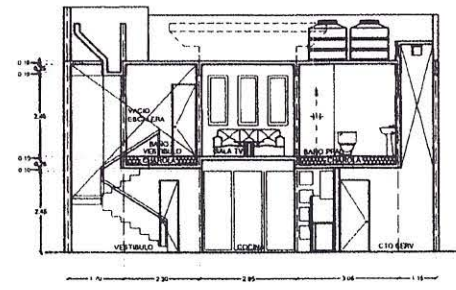
CORTE ESCALERA-BAÑOS-COCINA
