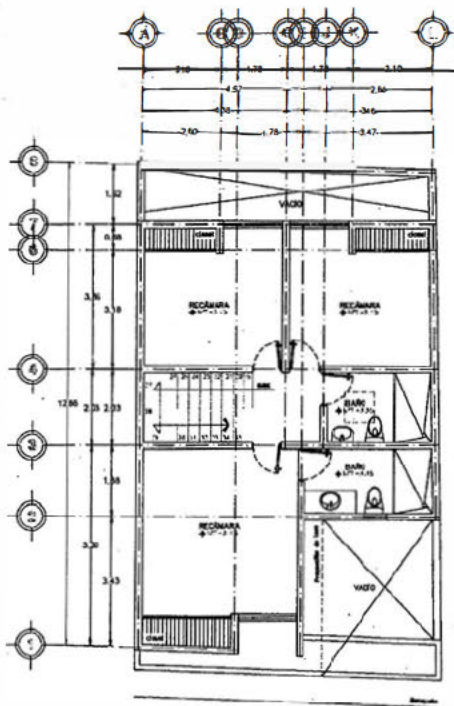
PRIMER NIVEL Estado Actual Escala 1:50
