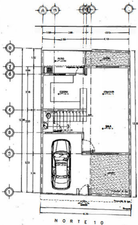
PLANTA BAJA Estado Actual Escala 1:50
