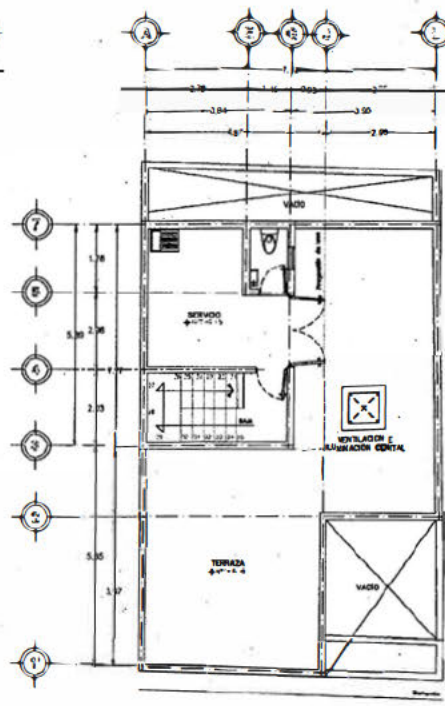
SEGUNDO NIVEL Estado Actual Escala 1:50
