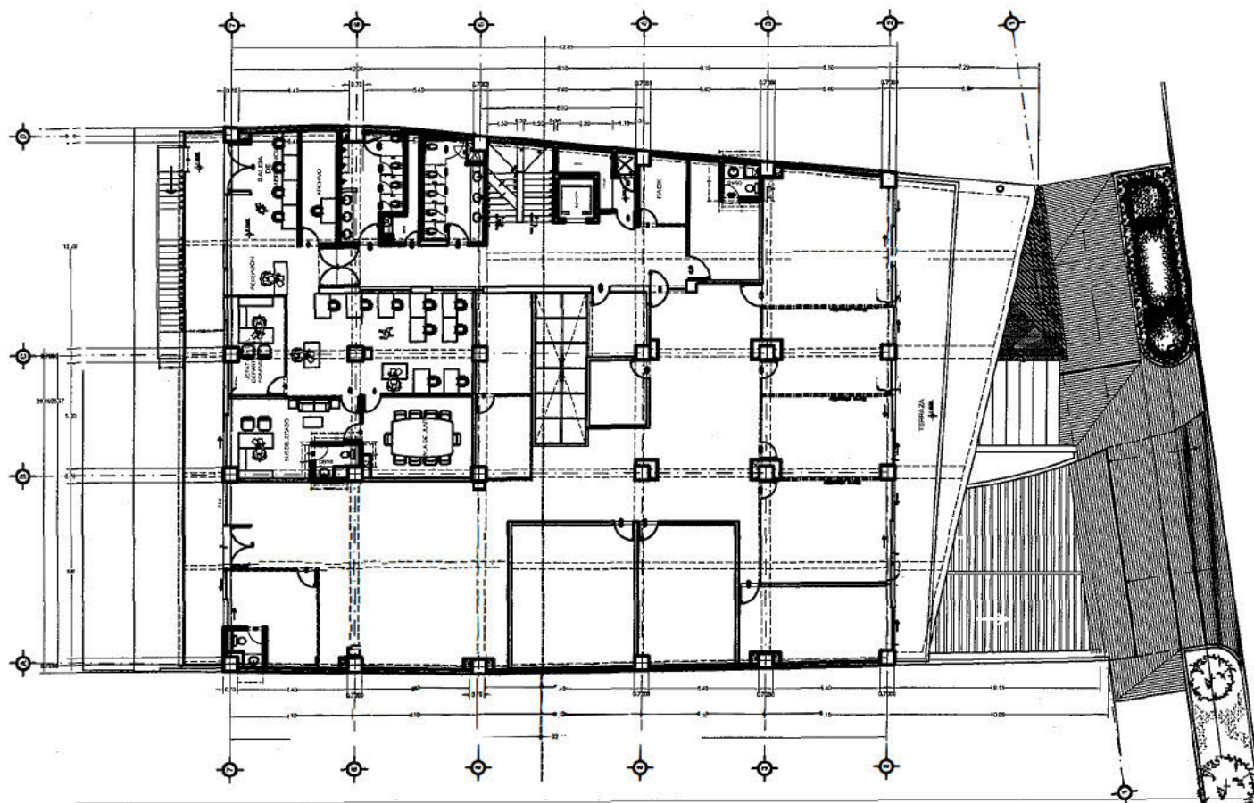
EDIFICIO SAT - ARQUITECTONICO PLANTA 3e NIVEL ÁREA TOTAL 3e NIVEL : 965.96 M2 ÁREA DE ARRENDAMIENTO : 160.69 M2
