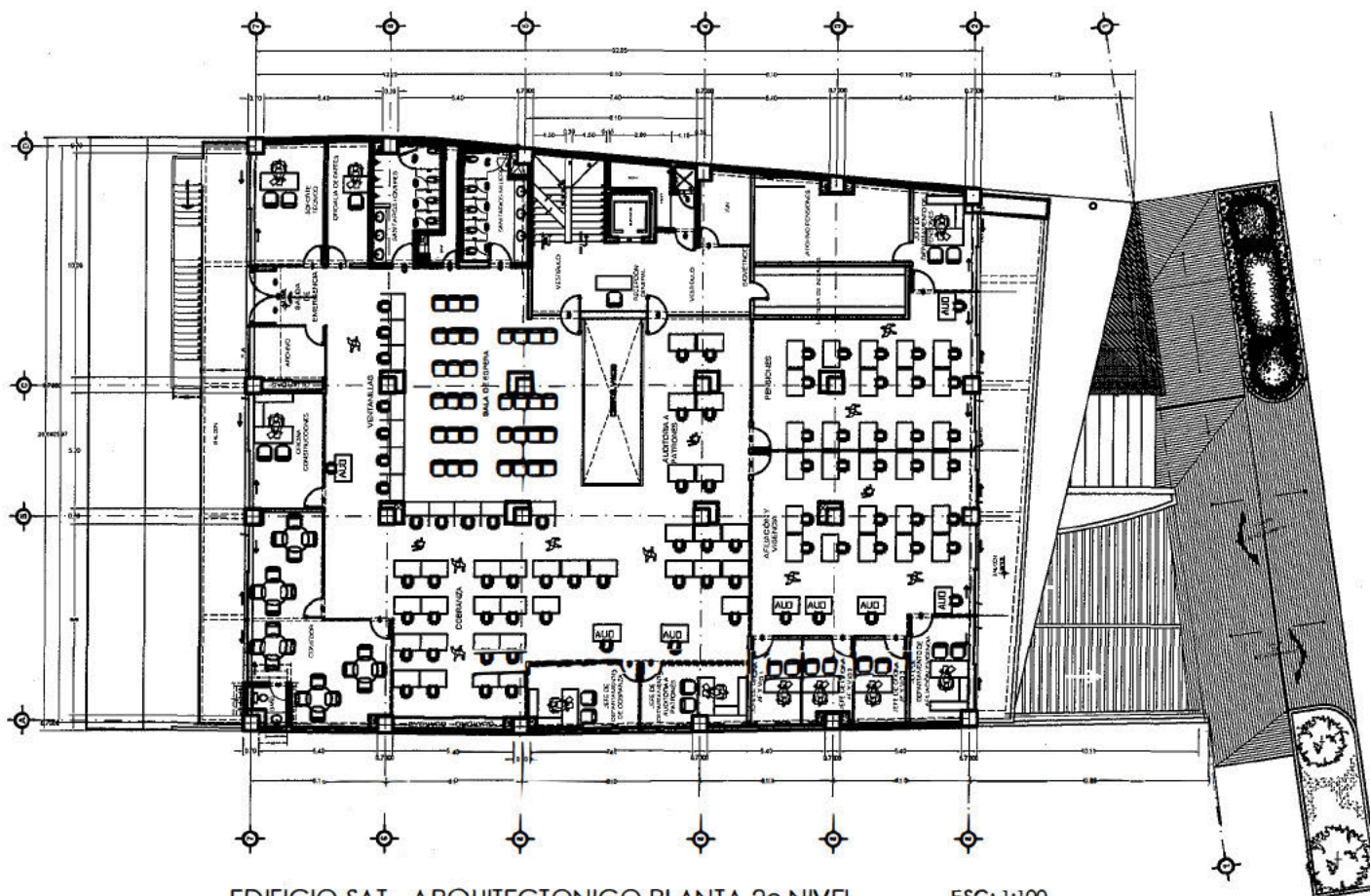
EDIFICIO SAT - ARQUITECTONICO PLANTA 2o NIVEL ÁREA TOTAL 2o NIVEL : 965.96 M2 ÁREA DE ARRENDAMIENTO : 965.96 M2
