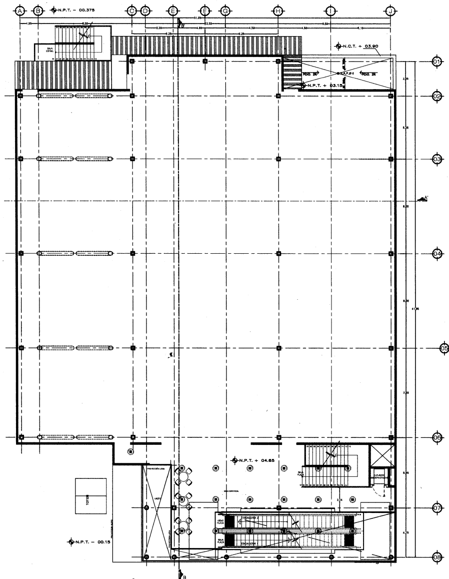
PLANO ARQUITECTÓNICO - PLANTA ALTA ÁREA : 1,268.01 M2
