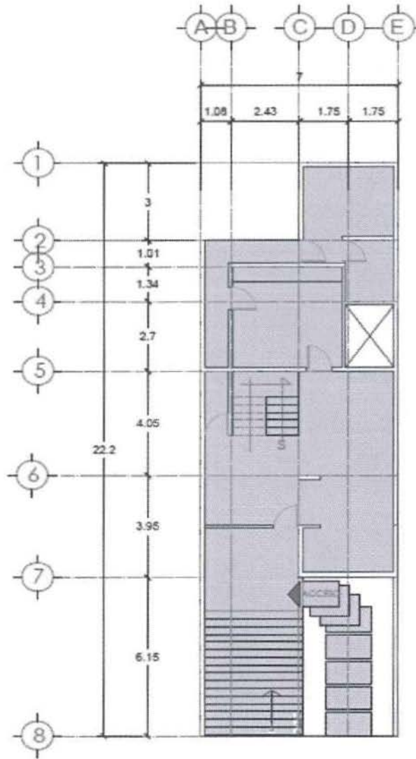
PLANTA ARQUITECTÓNICA
