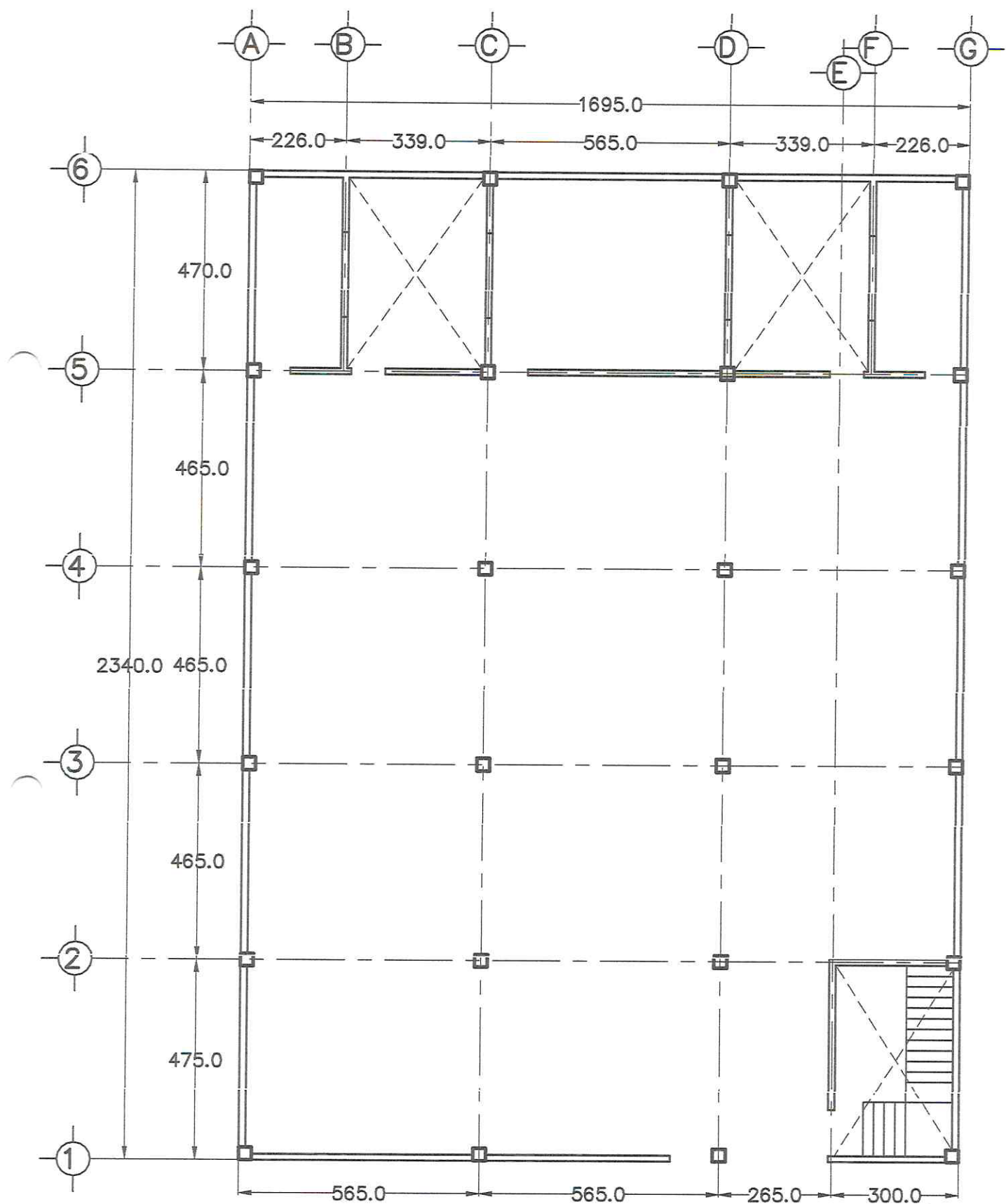
PLANTA BAJA
