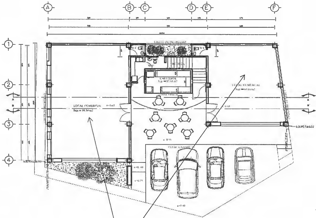
PLANTA ARQUITECTONICA BAJA
