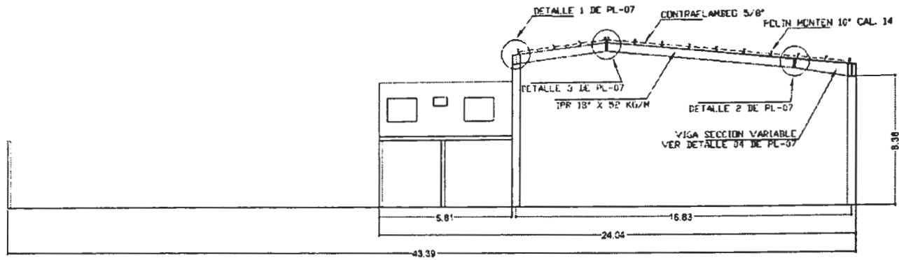
CORTE 2-2
