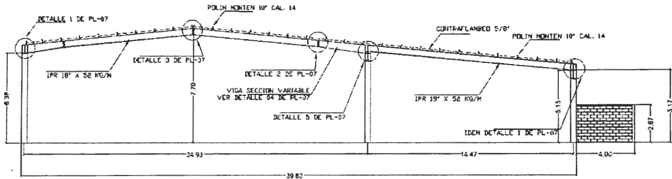
CORTE 1-1
