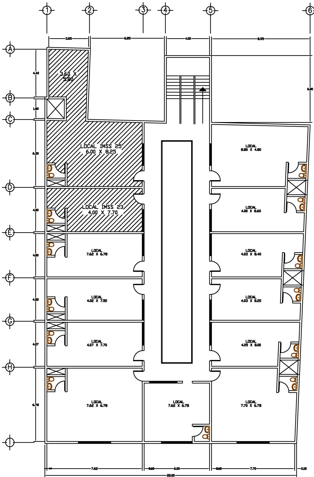
PLANTA ARQUITECTONICA ALTA
