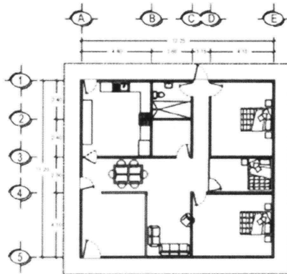
PLANTA ARQUITECTONICA ESC. 1:75
