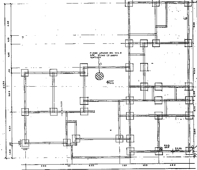
PLANO DE CIMENTACION ESC. 100
