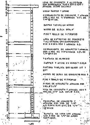
CORTE ESTRUCTURAL ESC. 150
