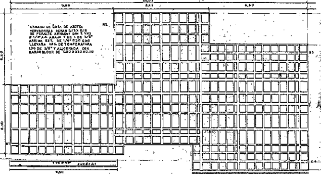
PLANO DE LOSAS (PLANTA ALTA) ESC. 100
