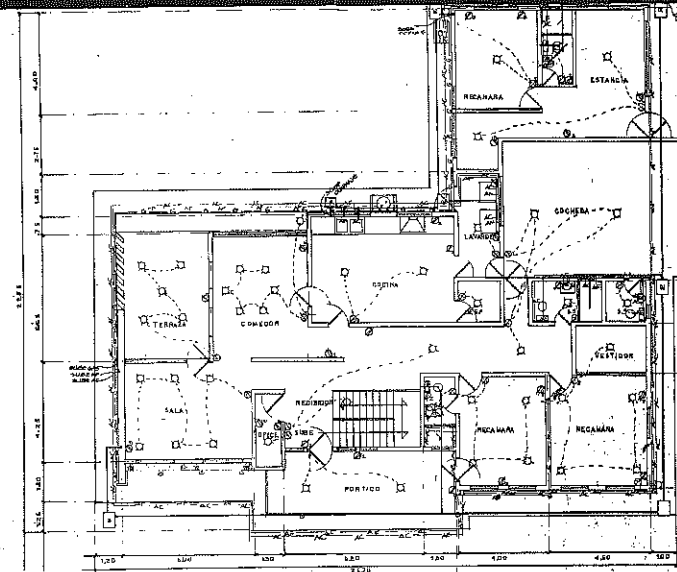
PLANTA ARQUITECTONICA BAJA ESC. 100 INSTALACIONES HIDRAULICAS SANITARIAS ELECTRICAS
