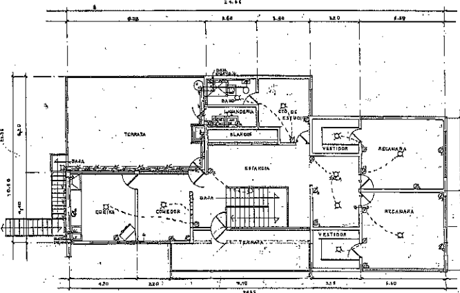
PLANTA ARQUITECTONICA ALTA ESC. 100 INSTALACIONES SANITARIAS HIDRAULICAS Y ELECTRICAS
