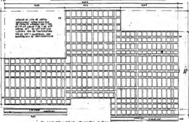
PLANO DE LOSAS (PLANTA ALTA) ESC.1/100
