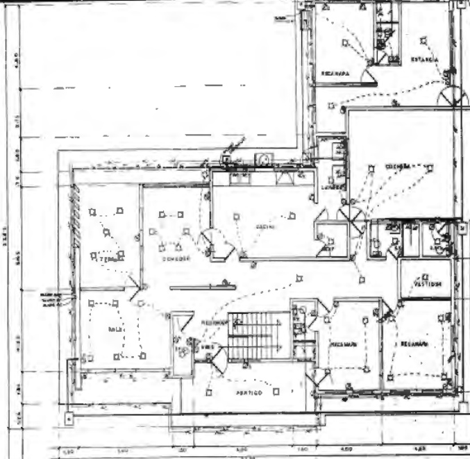
PLANTA ARQUITECTONICA BAJA ESC.1/100 INSTALACIONES HIDRAULICAS SANITARIAS ELECTRICAS
