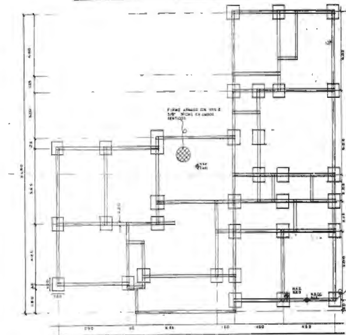
PLANO DE CIMENTACION ESC.1/100
