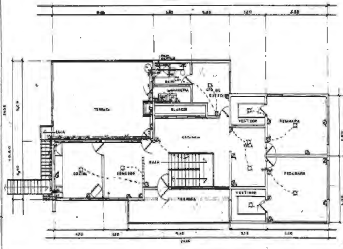
PLANTA ARQUITECTONICA ALTA ESC.1/100 INSTALACIONES SANITARIAS HIDRAULICAS Y ELECTRICAS
